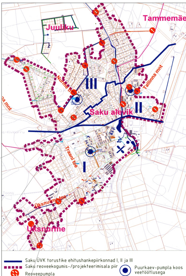
Saku aleviku ÜVK torustike ehitushanke piirkonnad: I Keskuse, II Kannikese, III Põhja-Saku
